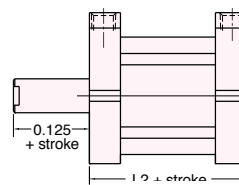
L2 + carrera Acción inversa AF-xRR-40x
